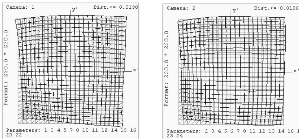
Rys.1. Wykresy dystorsji obrazu kamer którymi zrobiono zdjęcia bloku 7-68
